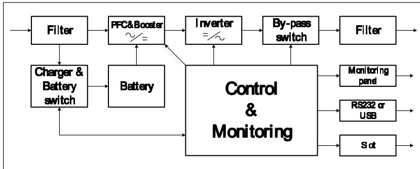
Fig.1. Schema a blocchi
