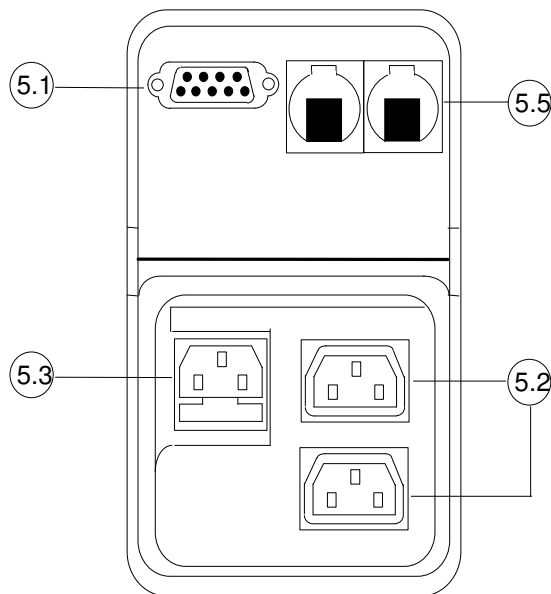
VISTA POSTERIORE EP800 S
